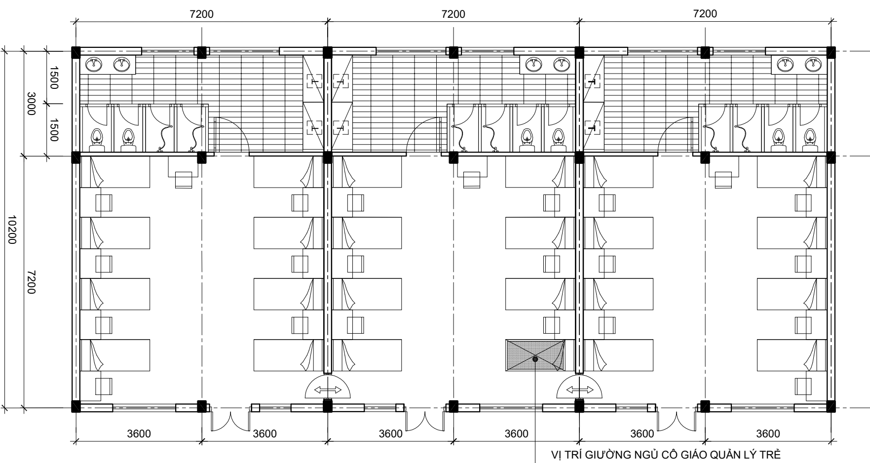
GỢI Ý GHEP 3 MODULE PHÒNG 8 HỌC SINH TIỂU HỌC (CÓ 1 CÔ GIÁO QUẢN LÝ GIÁM SÁT)
