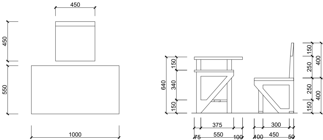
BÀN,GHẾ GIÁO VIÊN - KIỂU 2
