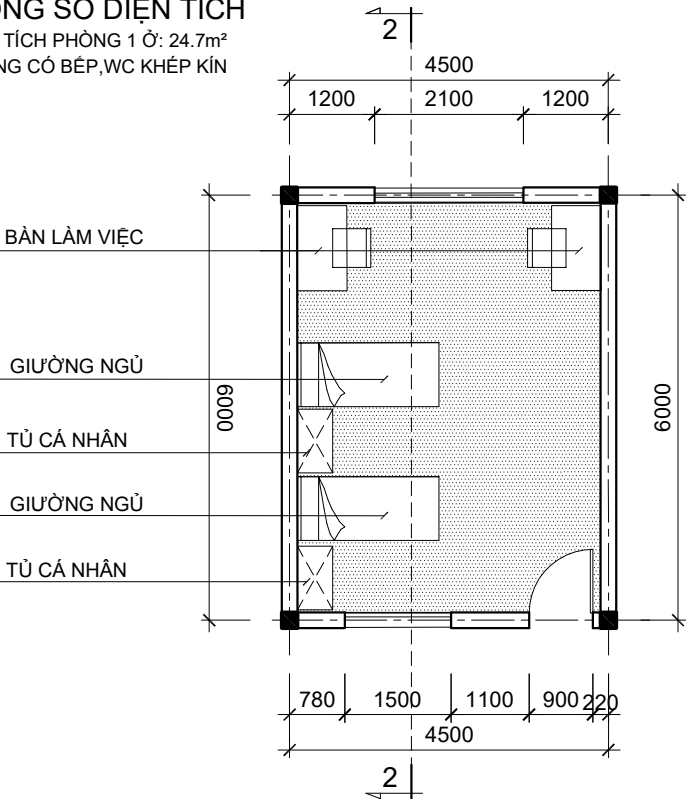
(LẮP GHÉP) QUY MÔ 10 GIÁO VIÊN - WC VÀ BẾP RIÊNG
