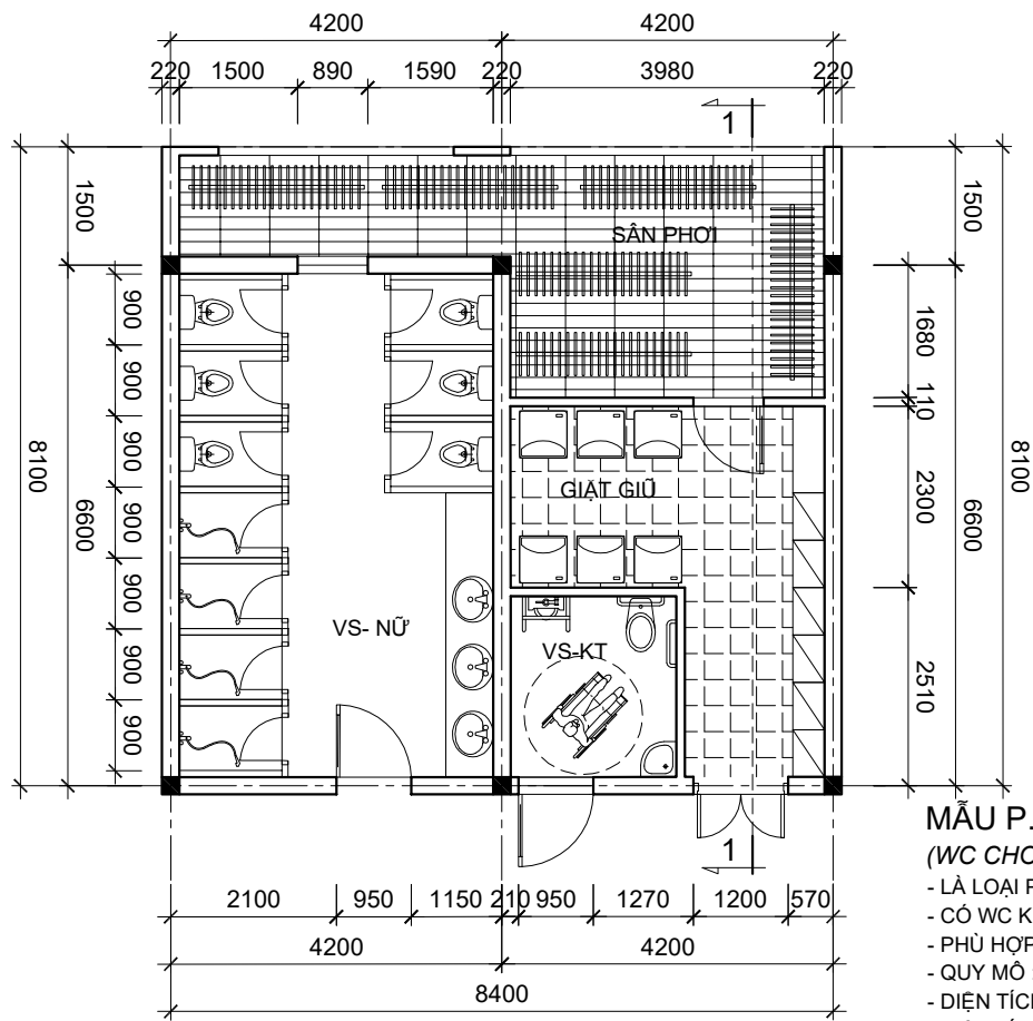
MẪU PHÒNG TẮM, VỆ SINH - 4A
