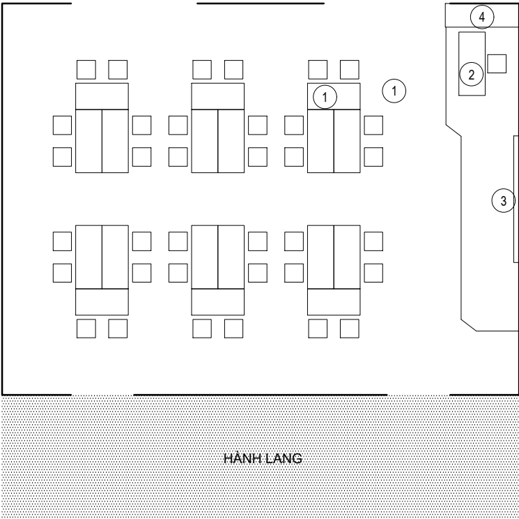
MẶT BẰNG PHÒNG HỌC BỐ TRÍ KIỂU HỌC NHÓM 6 NGƯỜI
