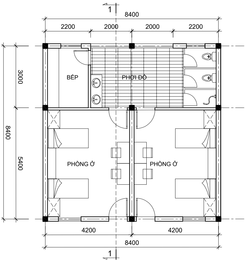
MẪU SỐ 1 - DIỆN TÍCH PHÒNG 1 Ở: 20.2m 2 - BẾP,WC, SÂN PHƠI (cho 2 module) : 23.6m 2 - VỆ SINH THIẾT KẾ THEO TIÊU CHUẨN HIỆN HÀNH (Xem chi tiết chung)
