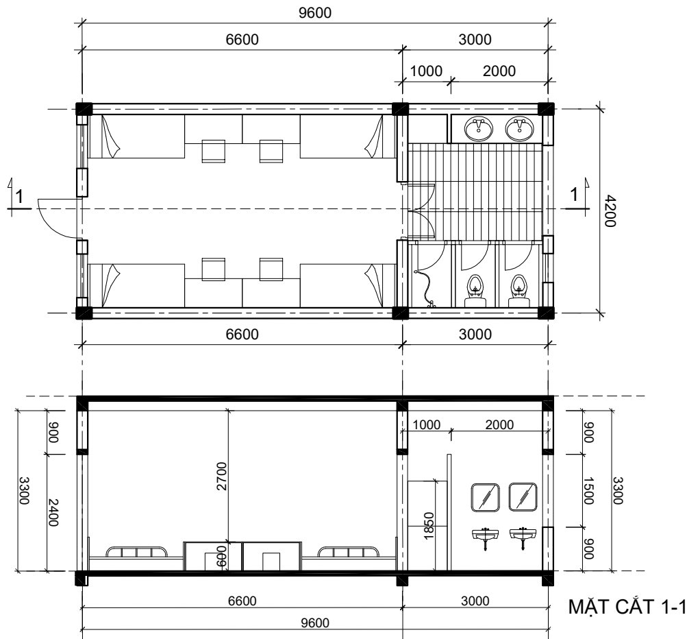
PHÒNG 4 HỌC SINH TIỂU HỌC (TH-4)
