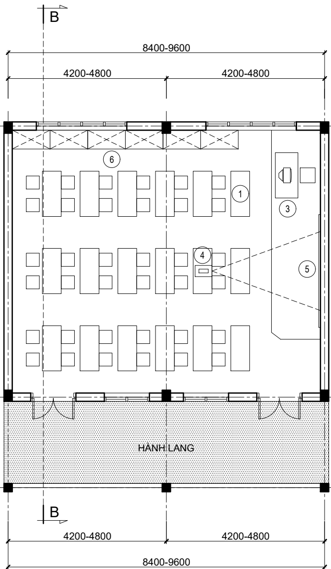
MẶT BẰNG PHÒNG HỌC BỘ MÔN NGOẠI NGỮ. (35 học sinh/lớp. Tiêu chuẩn diện tích: 1.5m 2 )
