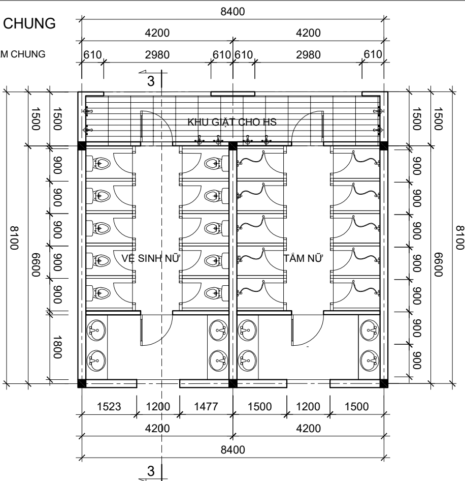
MẪU PHÒNG TẮM, VỆ SINH - 3B
