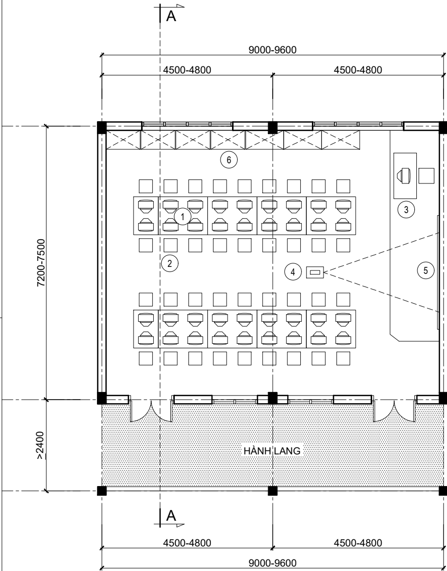
MẶT BẰNG PHÒNG HỌC BỘ MÔN TIN HỌC. (Tiêu chuẩn diện tích: 1.5m 2 )
