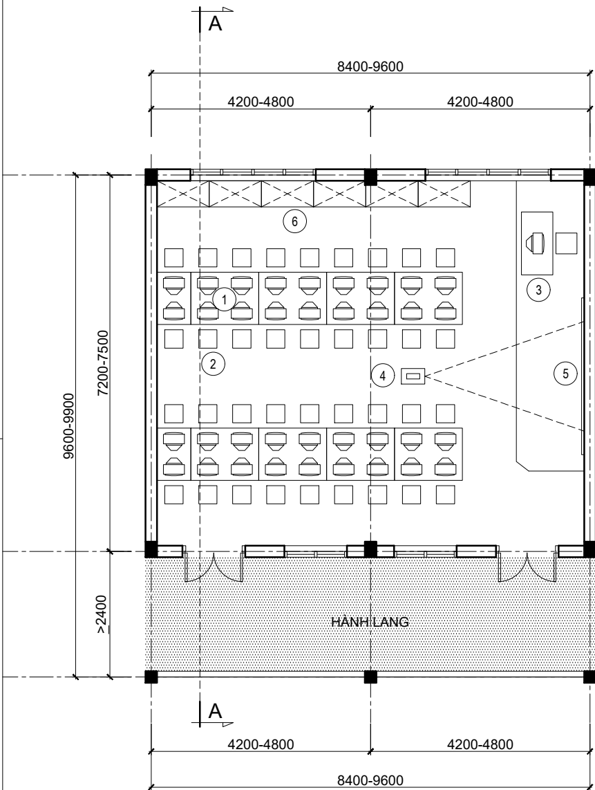
MẶT BẰNG PHÒNG HỌC BỘ MÔN TIN HỌC. (Tiêu chuẩn diện tích: 1.5m 2 )
