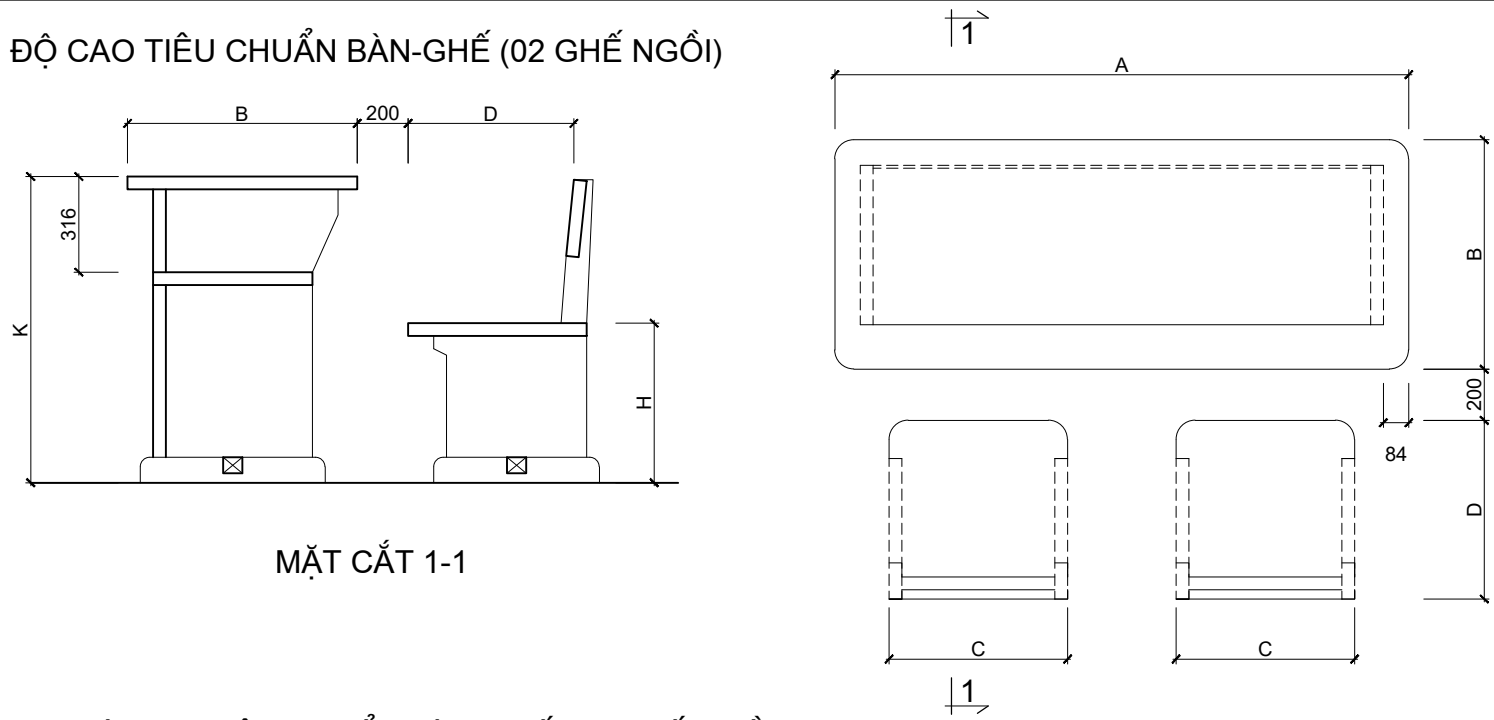
MẶT BẰNG BÀN VÀ GHẾ
