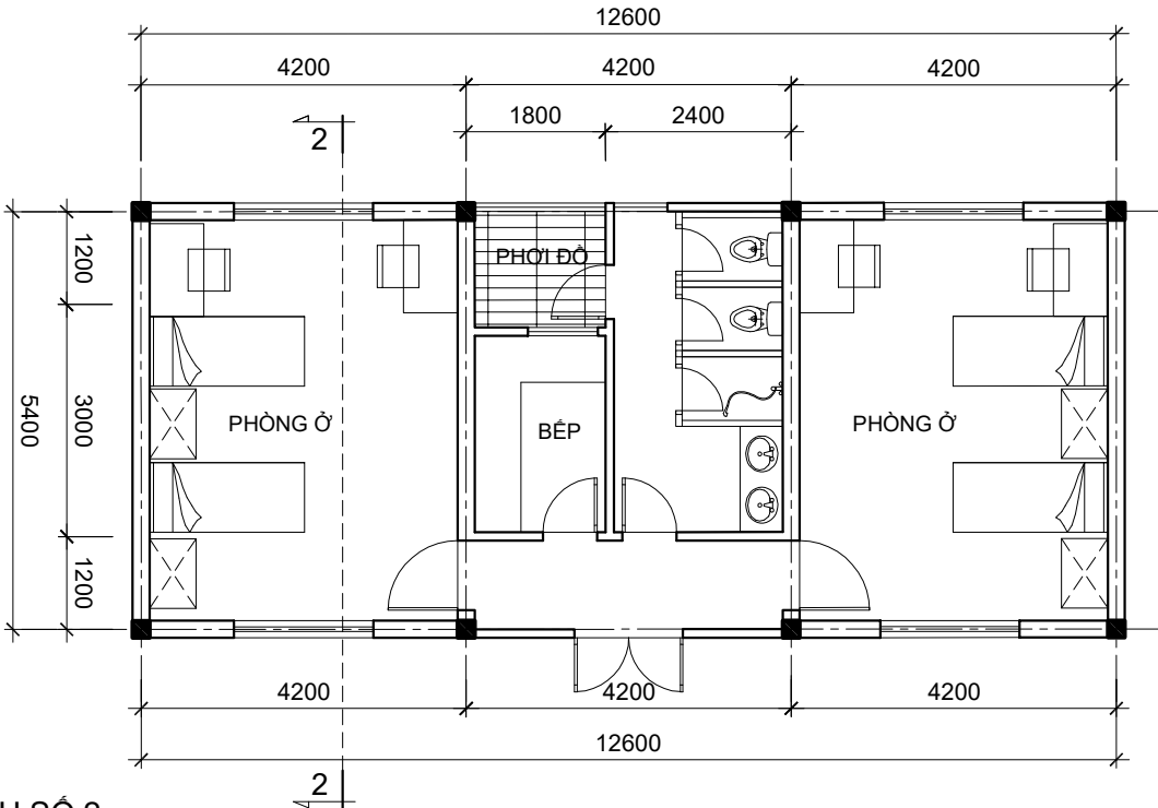
MẪU SỐ 2 - DIỆN TÍCH PHÒNG 1 Ở: 20.2m 2 - BẾP,WC, SÂN PHƠI (cho 2 module) : 16m 2 - VỆ SINH THIẾT KẾ THEO TIÊU CHUẨN HIỆN HÀNH (Xem chi tiết chung)
