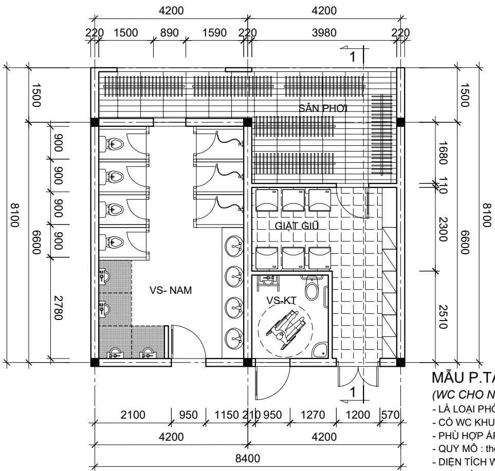
MẪU PHÒNG TẮM, VỆ SINH - 4B
