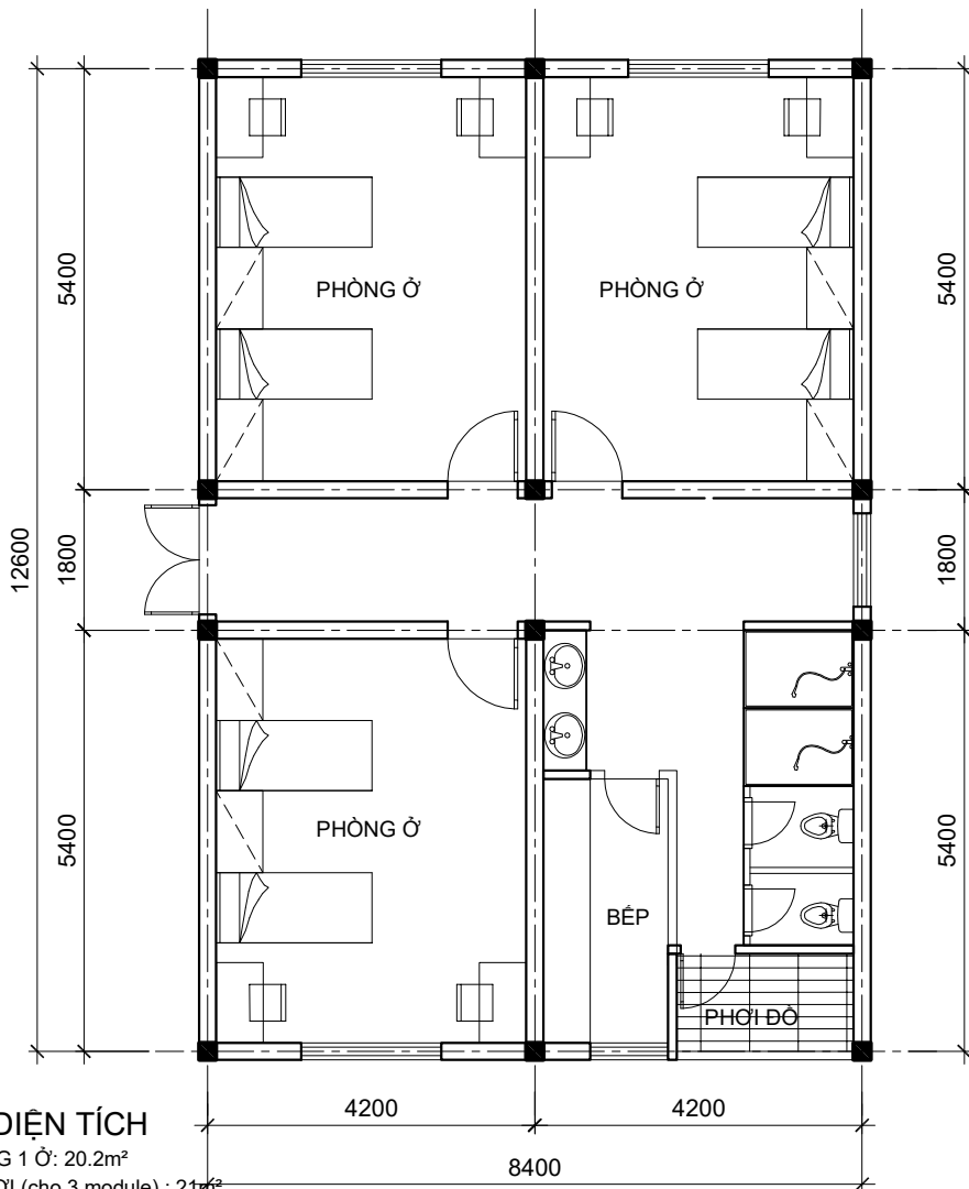
QUY MÔ 6 GIÁO VIÊN - CHUNG WC VÀ BẾP
