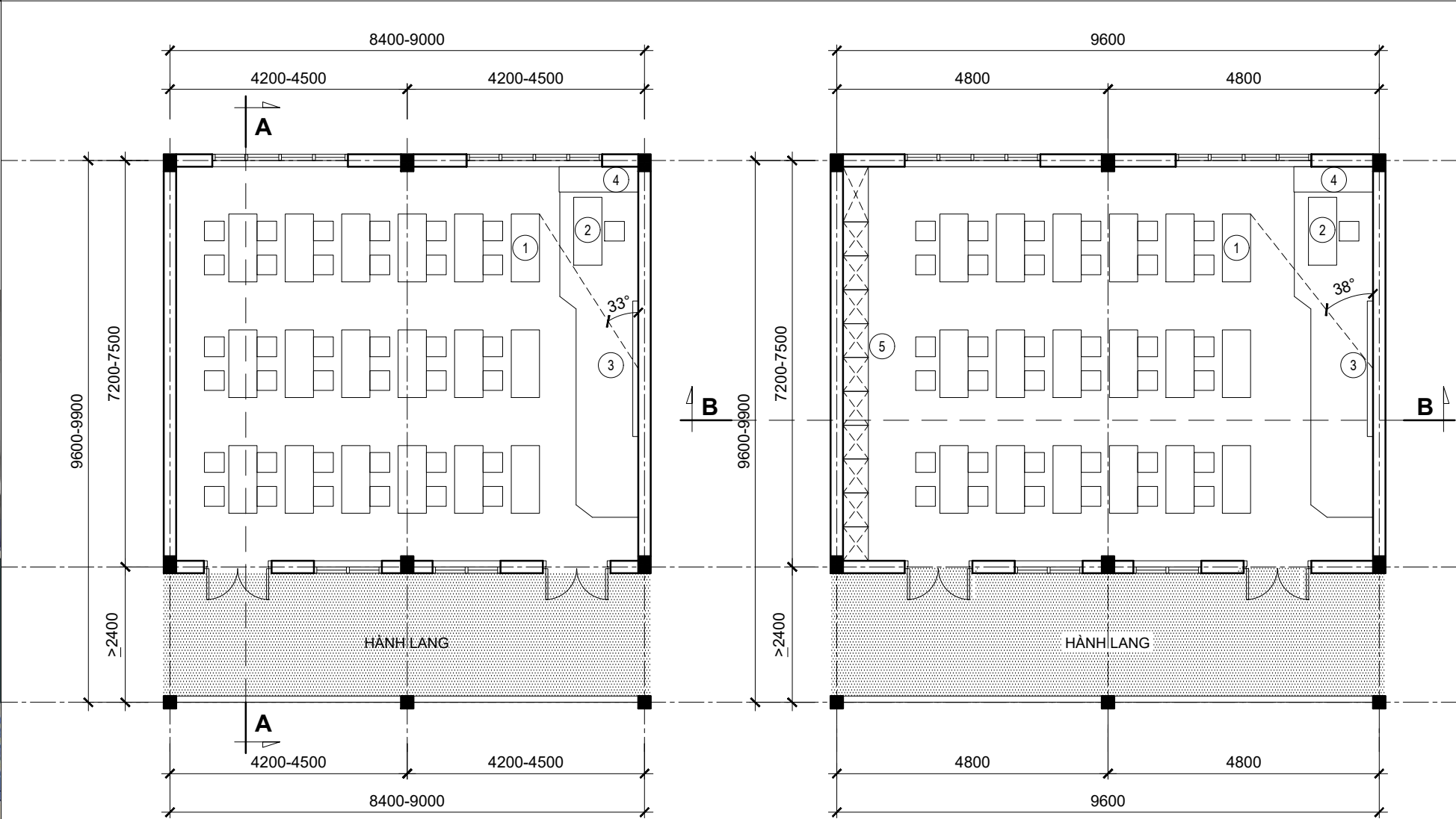
MẶT BẰNG PHÒNG HỌC KIỂU 1 (35 học sinh/lớp. Tiêu chuẩn diện tích: 1.5m 2 )
