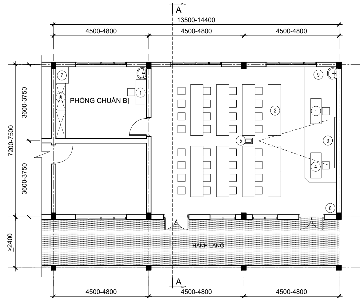
MẶT BẰNG PHÒNG HỌC BỘ MÔN KHOA HỌC CÔNG NGHỆ ÁP DỤNG CHO HỌC SINH CẤP TIỂU HỌC (Tiêu chuẩn diện tích: 1.85m²)
