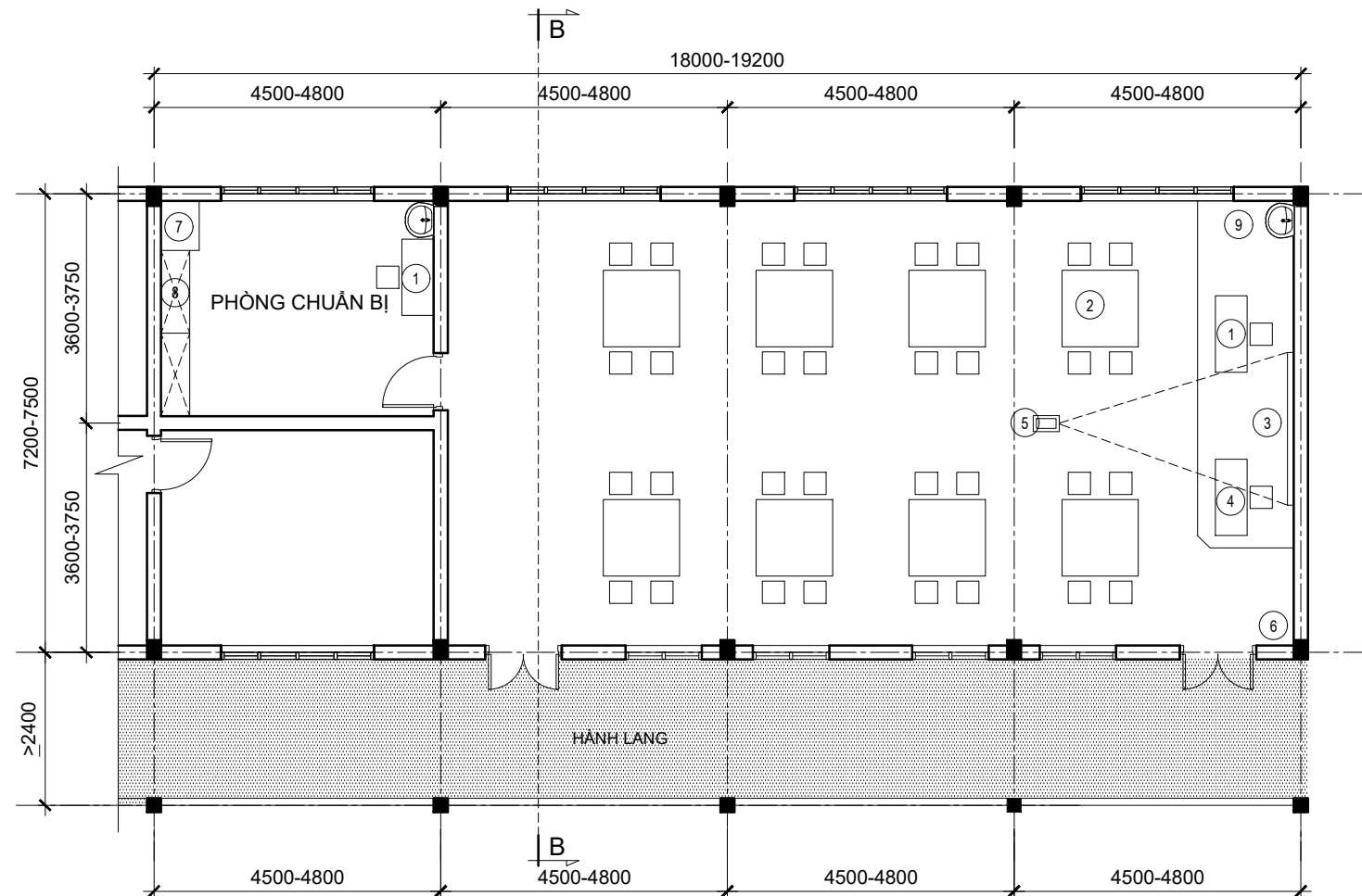
MẶT BẰNG PHÒNG HỌC BỘ MÔN CÔNG NGHỆ ÁP DỤNG CHO HỌC SINH CẤP THCS (Tiêu chuẩn diện tích: 2.25m²)
