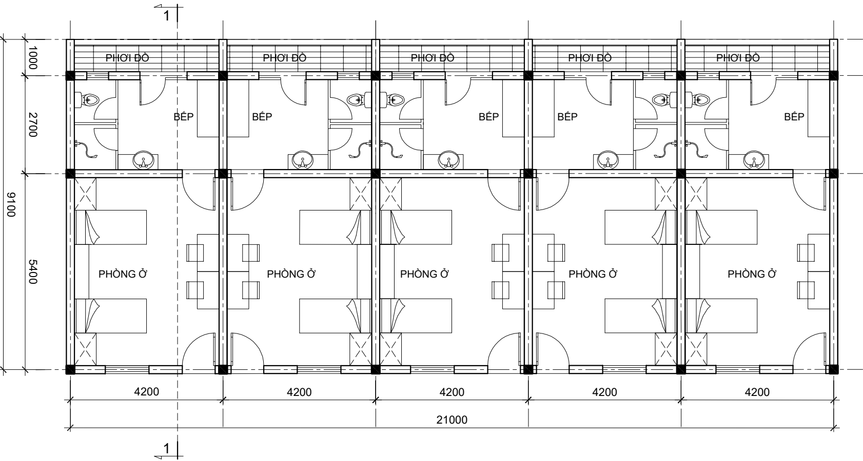
(LẮP GHÉP) QUY MÔ 10 GIÁO VIÊN - WC VÀ BẾP RIÊNG
