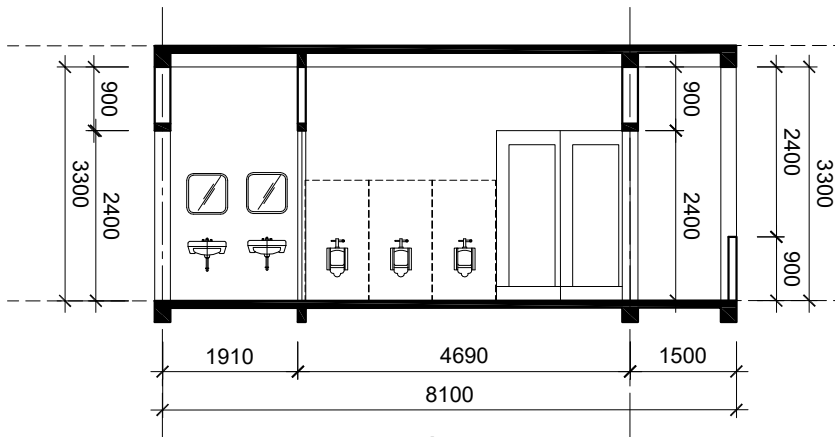
MẶT CẮT 2-2
