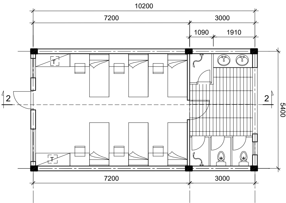
PHÒNG 6 HỌC SINH TIỂU HỌC (TH-6)
