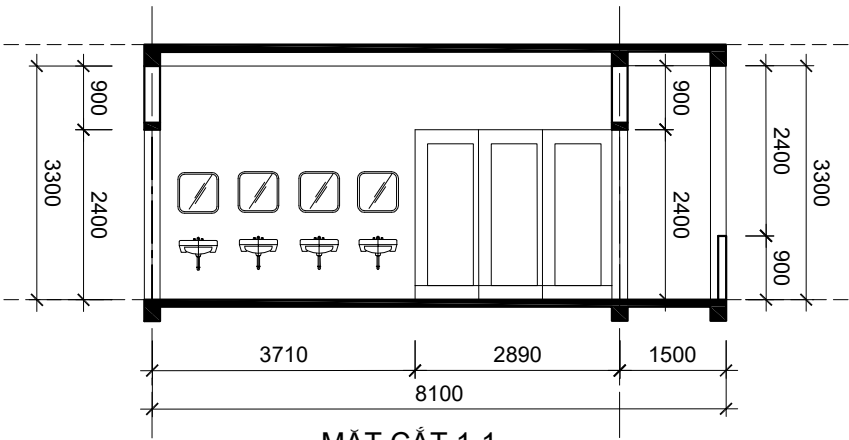
MẶT CẮT 1-1
