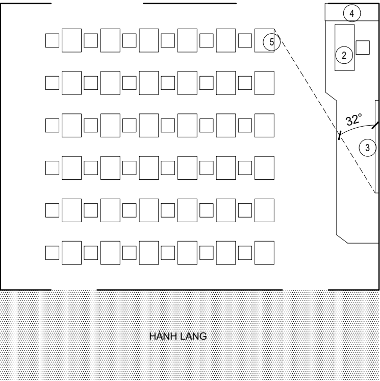
MẶT BẰNG PHÒNG HỌC BỐ TRÍ KIỂU HỌC NGỒI BÀN ĐƠN
