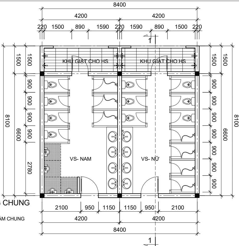
MẪU PHÒNG TẮM, VỆ SINH - 3
