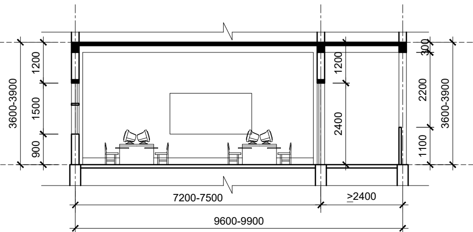
MẶT CẮT B - B
