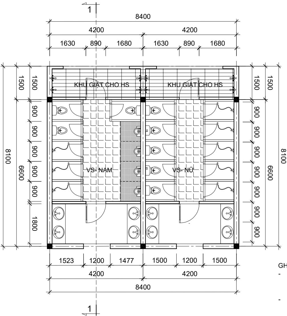
MẪU PHÒNG TẮM + WC DÙNG CHUNG
