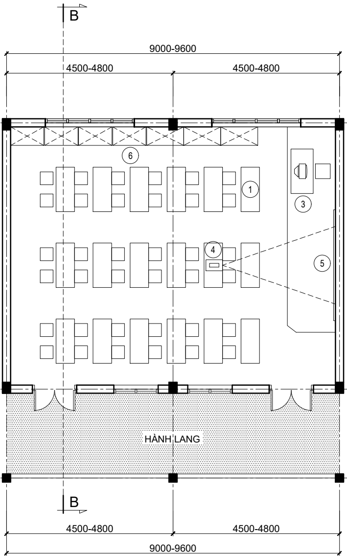
MẶT BẰNG PHÒNG HỌC BỘ MÔN NGOẠI NGỮ. (35 học sinh/lớp. Tiêu chuẩn diện tích: 1.5m 2 )
