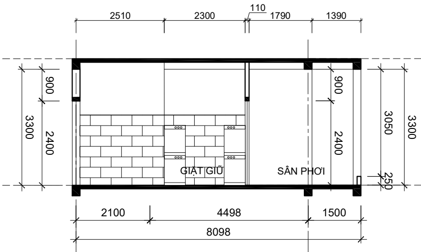
MẶT CẮT 1-1
