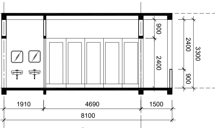
MẶT CẮT 3-3
