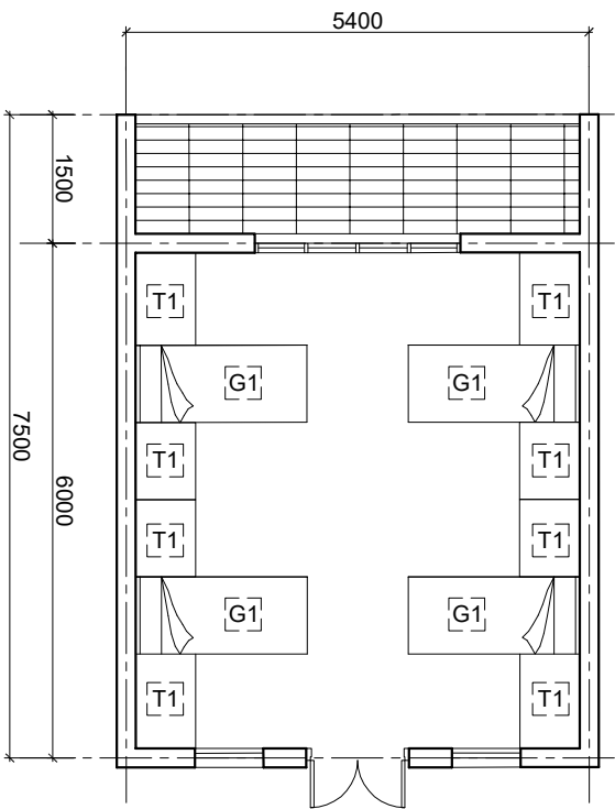
MẪU SỐ 2 - DIỆN TÍCH PHÒNG Ở: 32.4m 2 - DIỆN TÍCH BAN CÔNG: 8.1m 2
