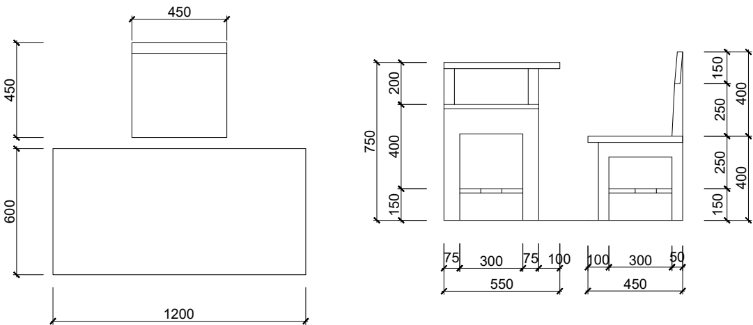
BÀN,GHẾ GIÁO VIÊN - KIỂU 2
