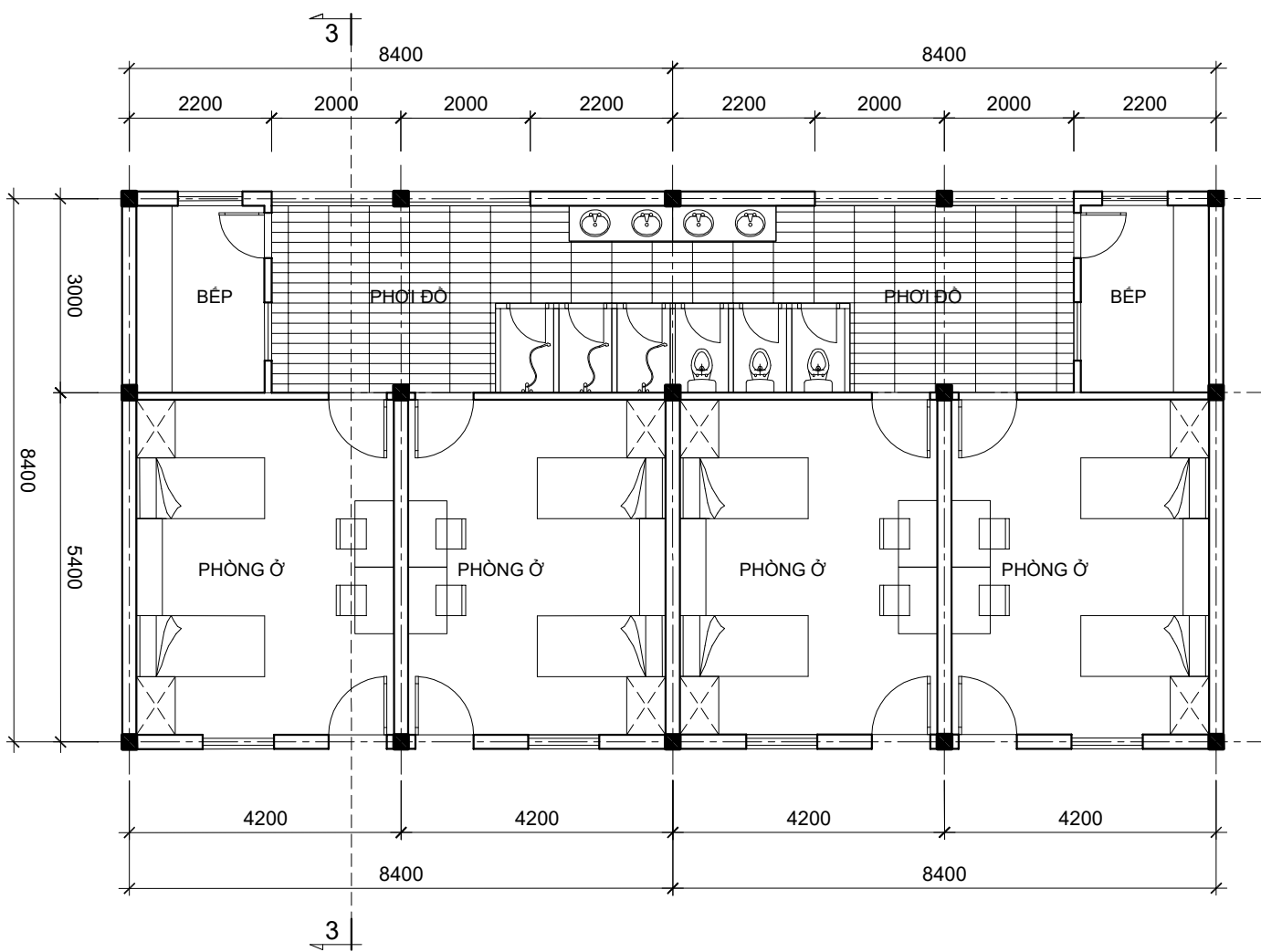
QUY MÔ 8 GIÁO VIÊN - CHUNG WC VÀ BẾP
