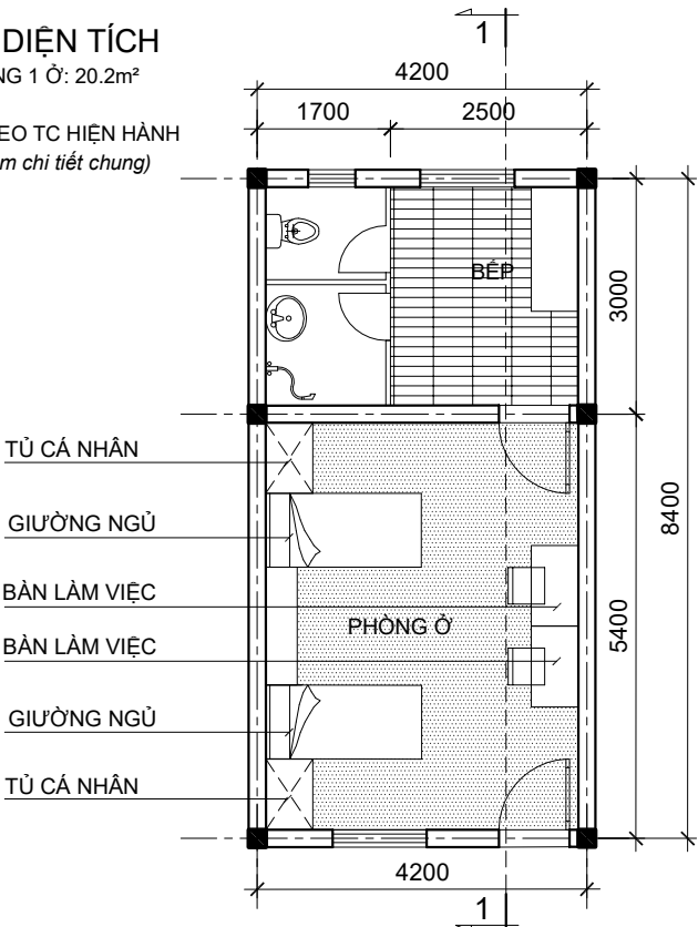
(LẮP GHÉP) QUY MÔ 10 GIÁO VIÊN - WC VÀ BẾP RIÊNG
