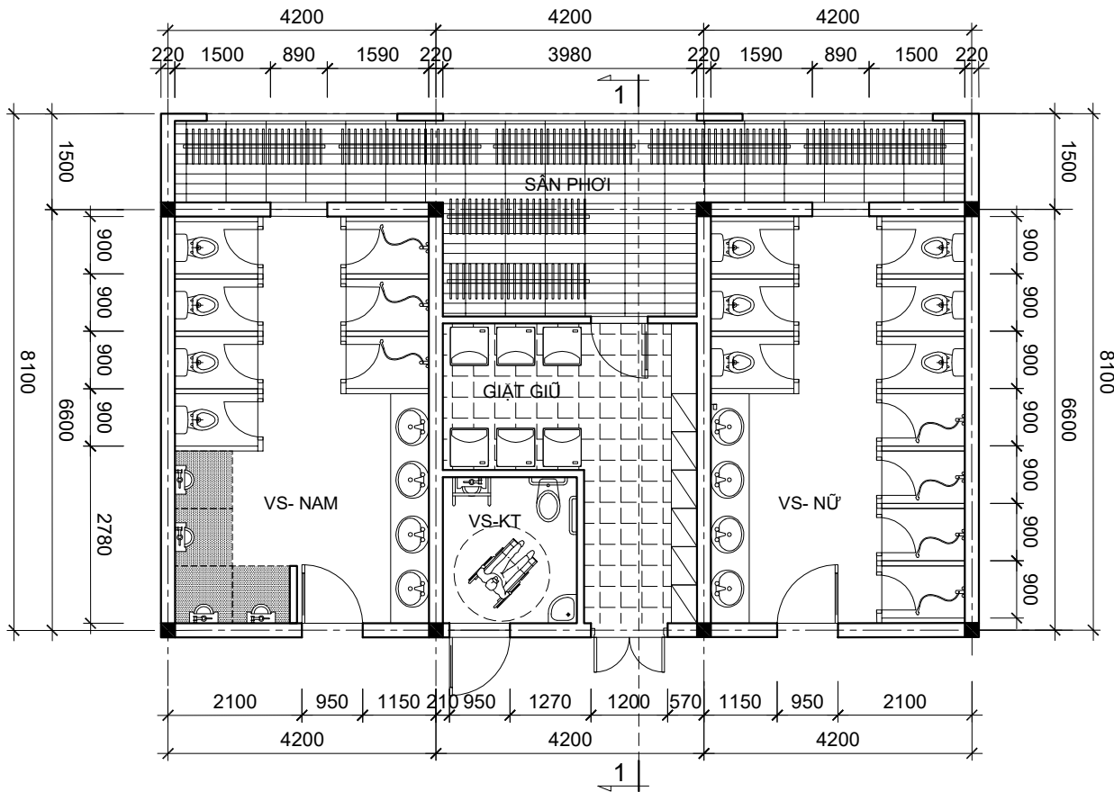
MẪU PHÒNG TẮM, VỆ SINH - 4
