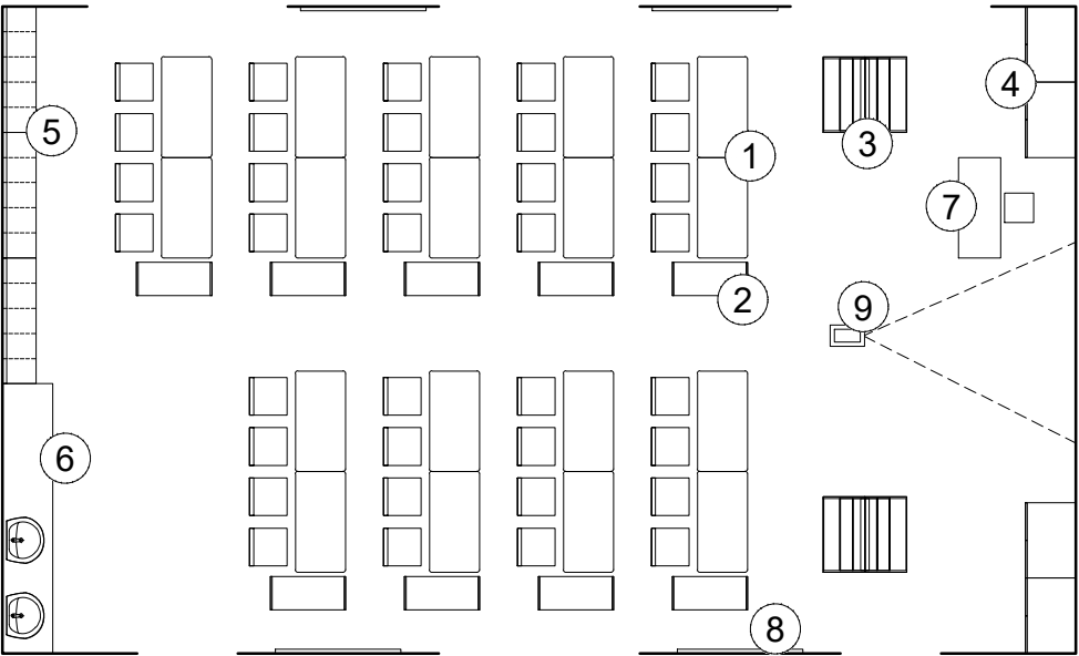
MẶT BẰNG PHÒNG HỌC STEM BỐ TRÍ KIỂU HỌC NHÓM 4 NGƯỜI
