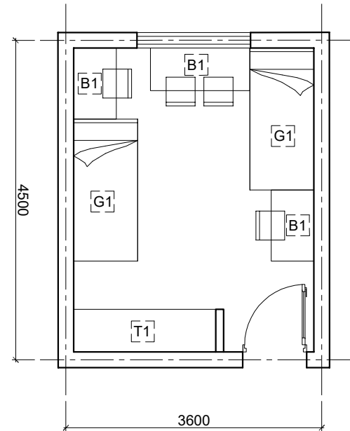
MẪU SỐ 1 - DIỆN TÍCH PHÒNG Ở: 28m 2
