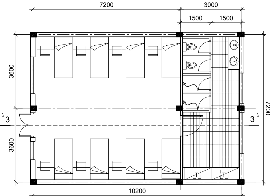
PHÒNG 8 HỌC SINH TIỂU HỌC (TH-8)
