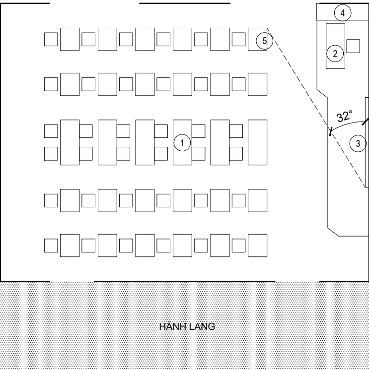
MẶT BẰNG PHÒNG HỌC BỐ TRÍ KIỂU HỌC KẾT HỢP BÀN ĐƠN VÀ BÀN ĐÔI
