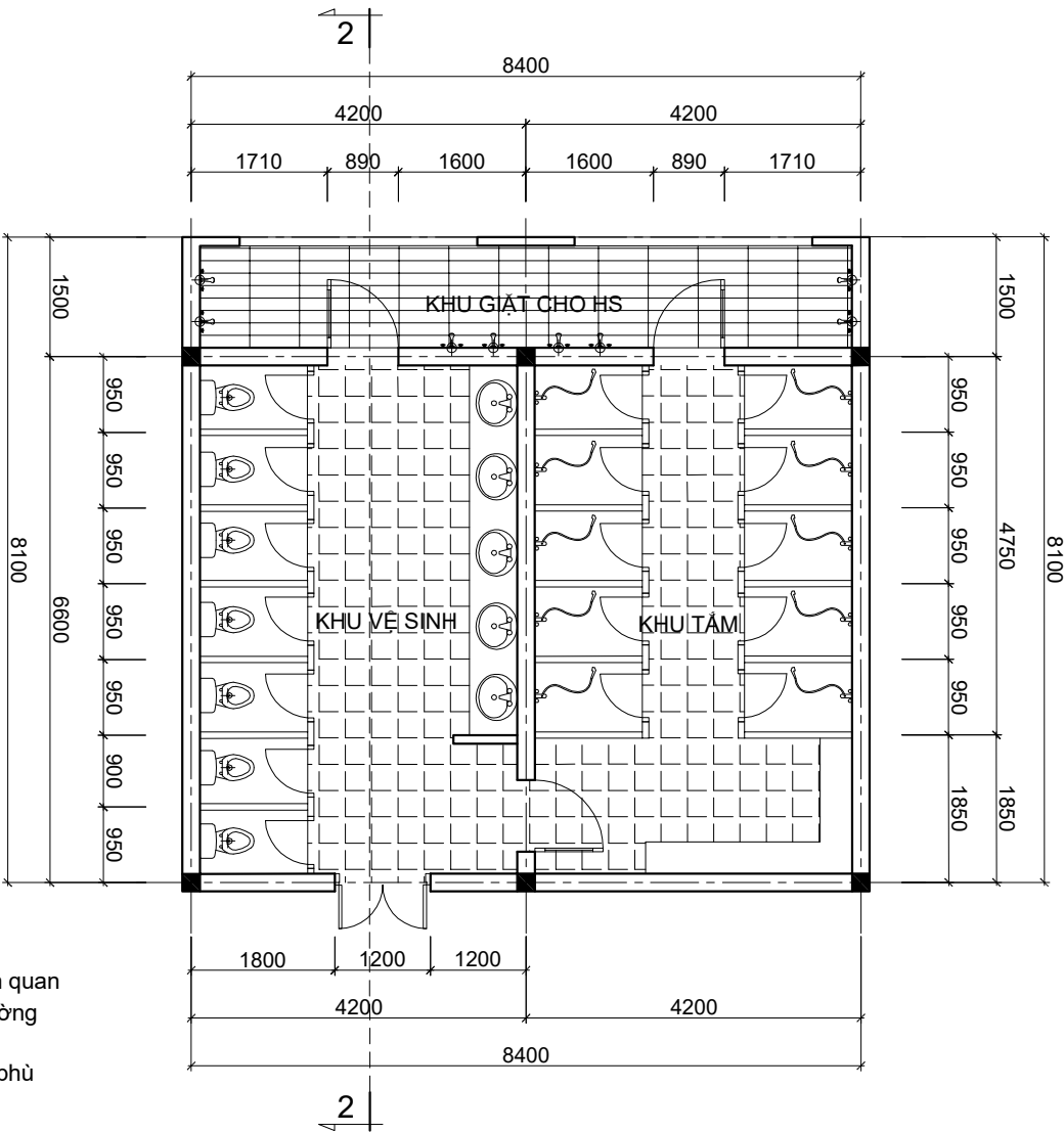
MẪU PHÒNG TẮM + WC DÙNG CHUNG
